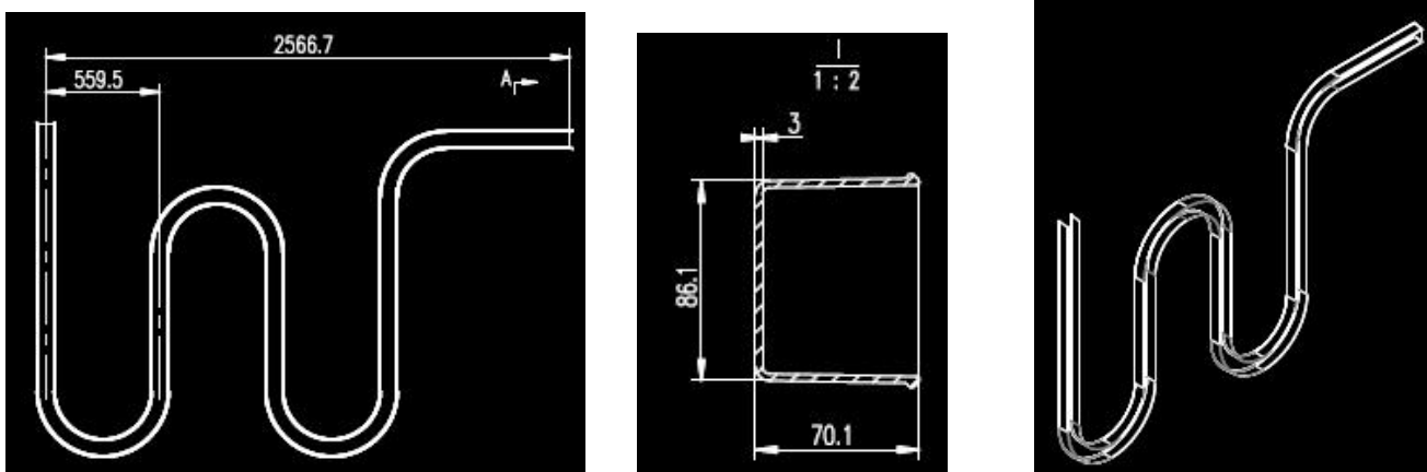
19 光纤槽 材质：SMC 比例：1:20
